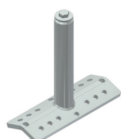
PALO BASE DOPPIA INCLINAZIONE 509 zincato a caldo
