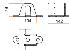
RAGNO INTERMEDIO 502 zincato a caldo
