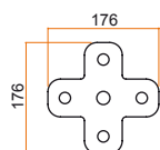
FARFALLA DI ESTREMITÀ 501 zincato a caldo
