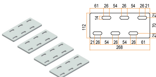
CONTROPIASTRA PER PIASTRA RIPARTITRICE 405A n. 4 pezzi zincato
