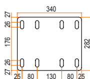
CONTROPIASTRA PER BASE ALLARGATA PIANA 532 zincato
