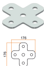
FARFALLA DI ESTREMITÀ 501 zincato a caldo
