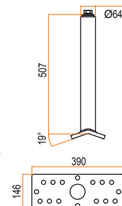
PALO BASE DOPPIA INCLINAZIONE 506 zincato a caldo
