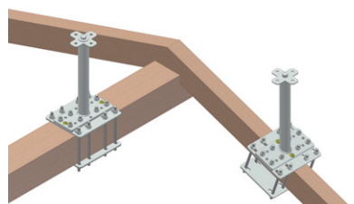
Staffaggio con base allargata, barre filettate e contropiastra, o con profili di riscontro
