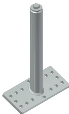
PALO BASE INCLINATA 504 zincato a caldo
