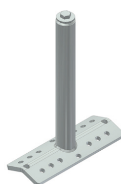
PALO BASE DOPPIA INCLINAZIONE 506 zincato a caldo
