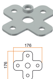
FARFALLA ROTANTE 501A zincato a caldo
