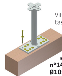
Staffaggio con base allargata, barre filettate e contropiastra, o con profili di riscontro
