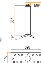
PALO BASE DOPPIA INCLINAZIONE 509 zincato a caldo
