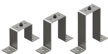
DISTANZIALE 392 zincato H 100 mm 392A zincato H 150 mm 392B zincato H 200 mm
