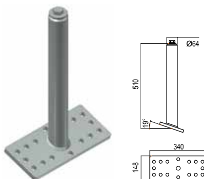
PALO BASE INCLINATA 504-50 zincato a caldo 504-50C inox
