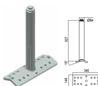
PALO BASE DOPPIA INCLINAZIONE 506-50 zincato a caldo 506-50C inox
