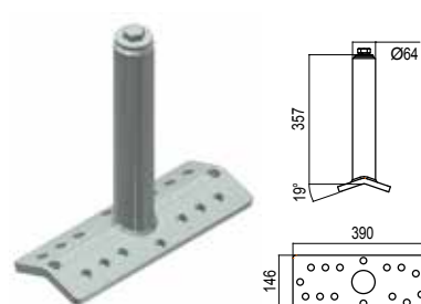
PALO BASE DOPPIA INCLINAZIONE 506-35 zincato a caldo 506-35C inox
