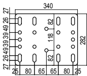
BASE ALLARGATA PIANA 531 zincato
