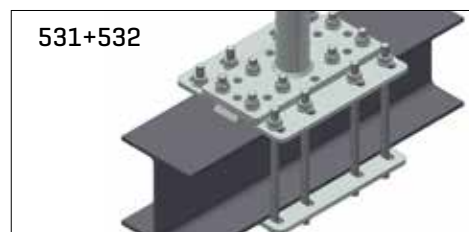
Staffaggio con base allargata, barre filettate e contropiastre, o profili di riscontro [vedi NOTA ]
