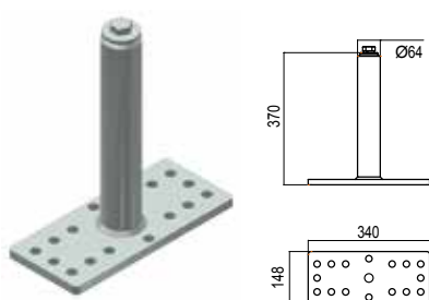
PALO BASE PIANA 503-35 zincato a caldo 503-35C inox
