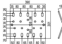
BASE ALLARGATA DOPPIA INCLINAZIONE 533 zincato
