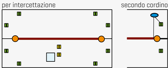
Linea vita unidirezionale a campata unica
