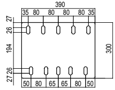
CONTROPIASTRA PER BASE ALLARGATA DOPPIA INCLINAZIONE 534 zincato
