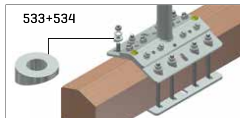
Nello staffaggio su travi inclinate, utilizzare la rondella inclinata art. 419D.
