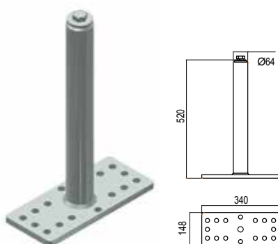
PALO BASE PIANA 503-50 zincato a caldo 503-50C inox
