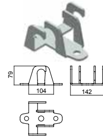
RAGNO INTERMEDIO 502 zincato a caldo 502C inox
