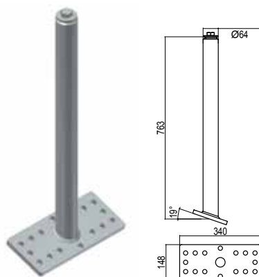
PALO BASE INCLINATA 504-75 zincato a caldo 504-75C inox
