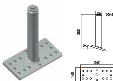
PALO BASE INCLINATA 504-35 zincato a caldo 504-35C inox
