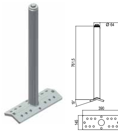
PALO BASE DOPPIA INCLINAZIONE 506-75 zincato a caldo 506-75C inox
