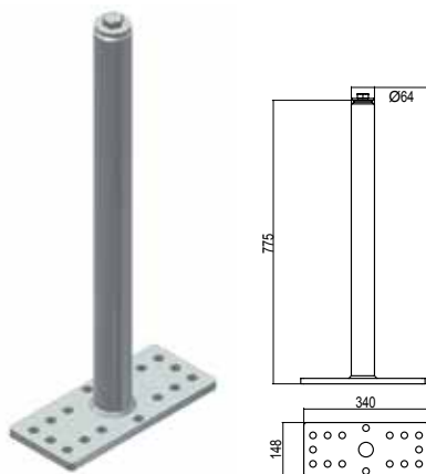
PALO BASE PIANA 503-75 zincato a caldo 503-75C inox
