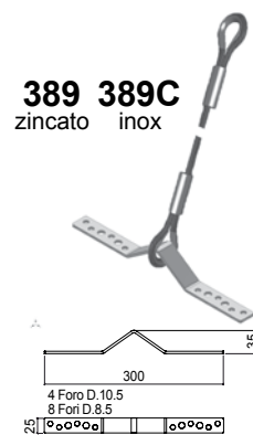
Ancoraggio con fune
