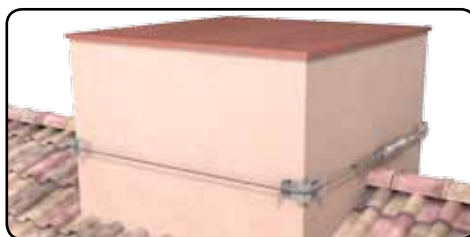
Caso di linea vita a parete su 4 lati: ancoraggi 601H-601L.
