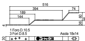
Piastra ripartitrice di carico
