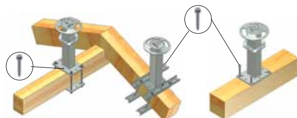
Staffaggio con barre filettate, contropiastre o profili di riscontro (vedi NOTA )
