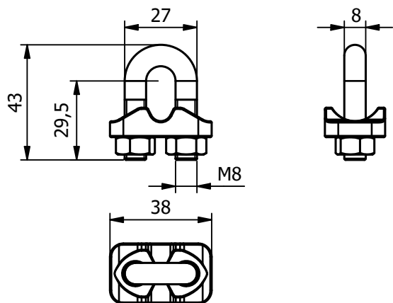
Codice 434B: Morsetto
