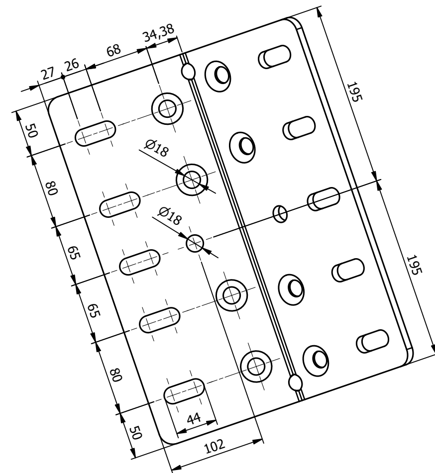
Vista B-B
