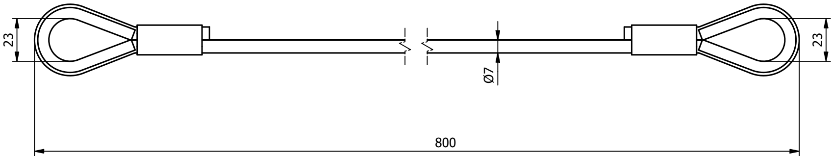
Dimensioni fune codice 389-02-7C
