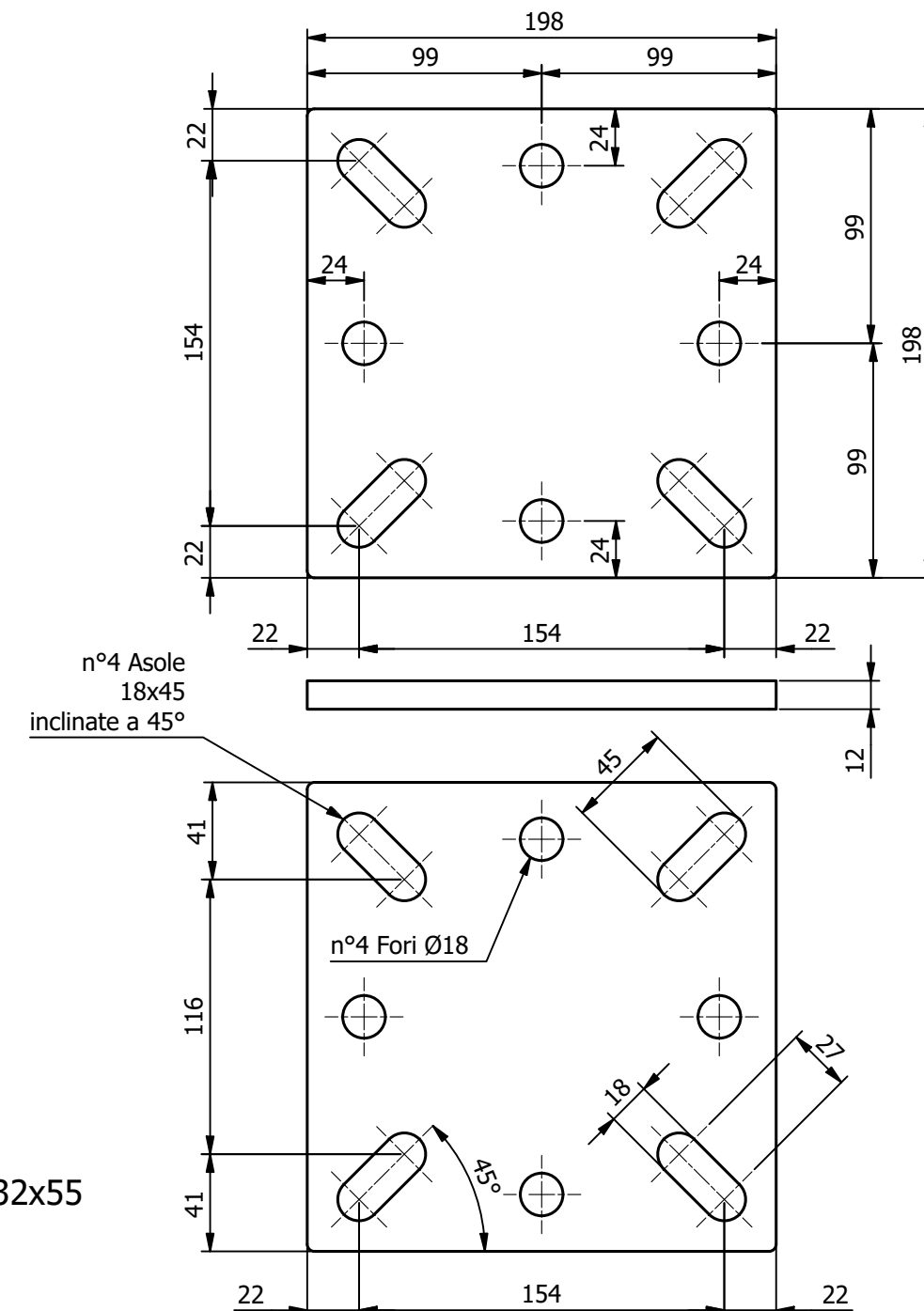
Rappresentazione base piana (cod. 908C) con posizione dei fori Scala 1:3
