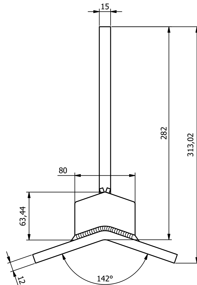
Rappresentazione marcatura Scala 1:1
