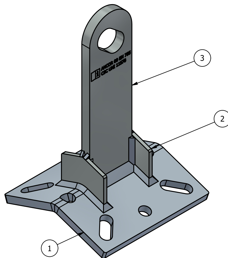
Rappresentazione marcatura Scala 1:1
