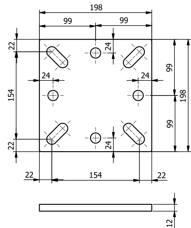
Rappresentazione base piana (cod. 908C) con posizione dei fori Scala 1:4
