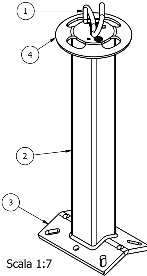
n°4 Asole 18x45 n°4 fori Ø 18
