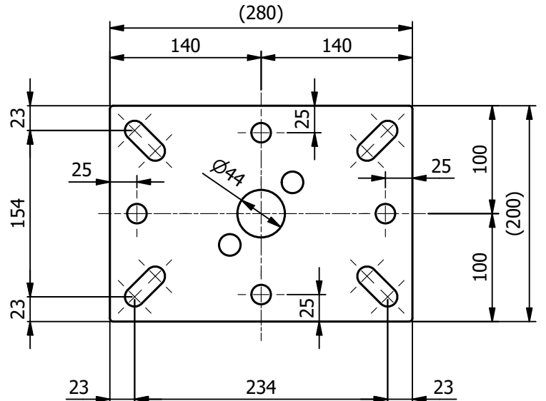
Rappresentazione base piana (cod. 902A.2) con posizione fori ed asole (scala 1:5)
