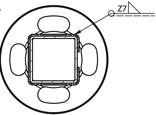
Sez. A-A
