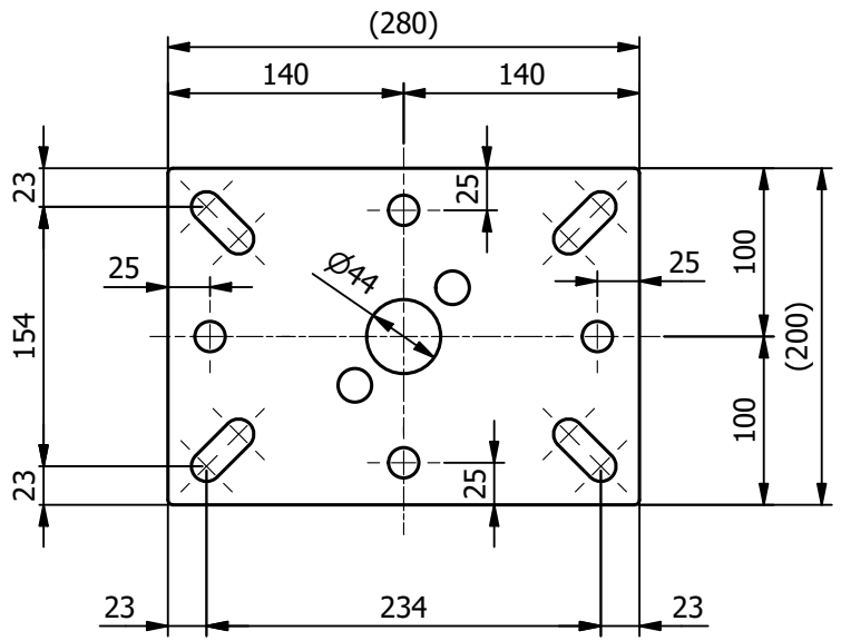
Rappresentazione base piana (cod. 902A.2) con posizione fori ed asole (scala 1:5)
