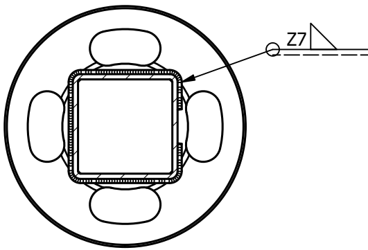
Sez. A-A
