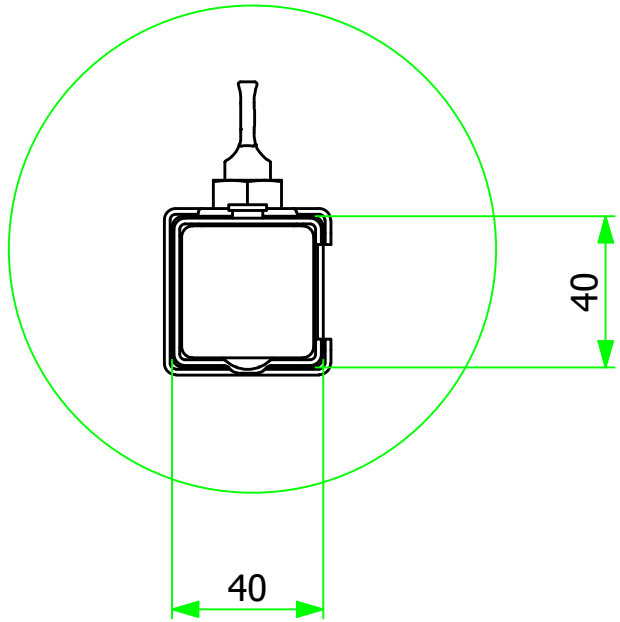
Dettaglio "A" Scala 1 : 2
