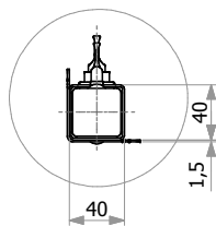
Dettaglio A Scala 1 : 3
