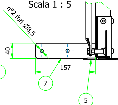
Dettaglio E Scala 1 : 5
