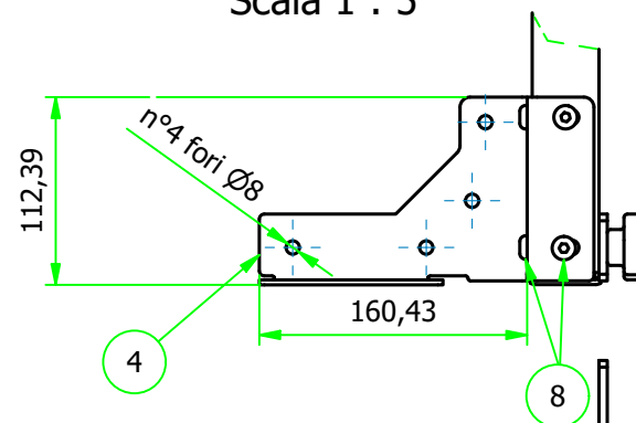
Dettaglio D Scala 1 : 5
