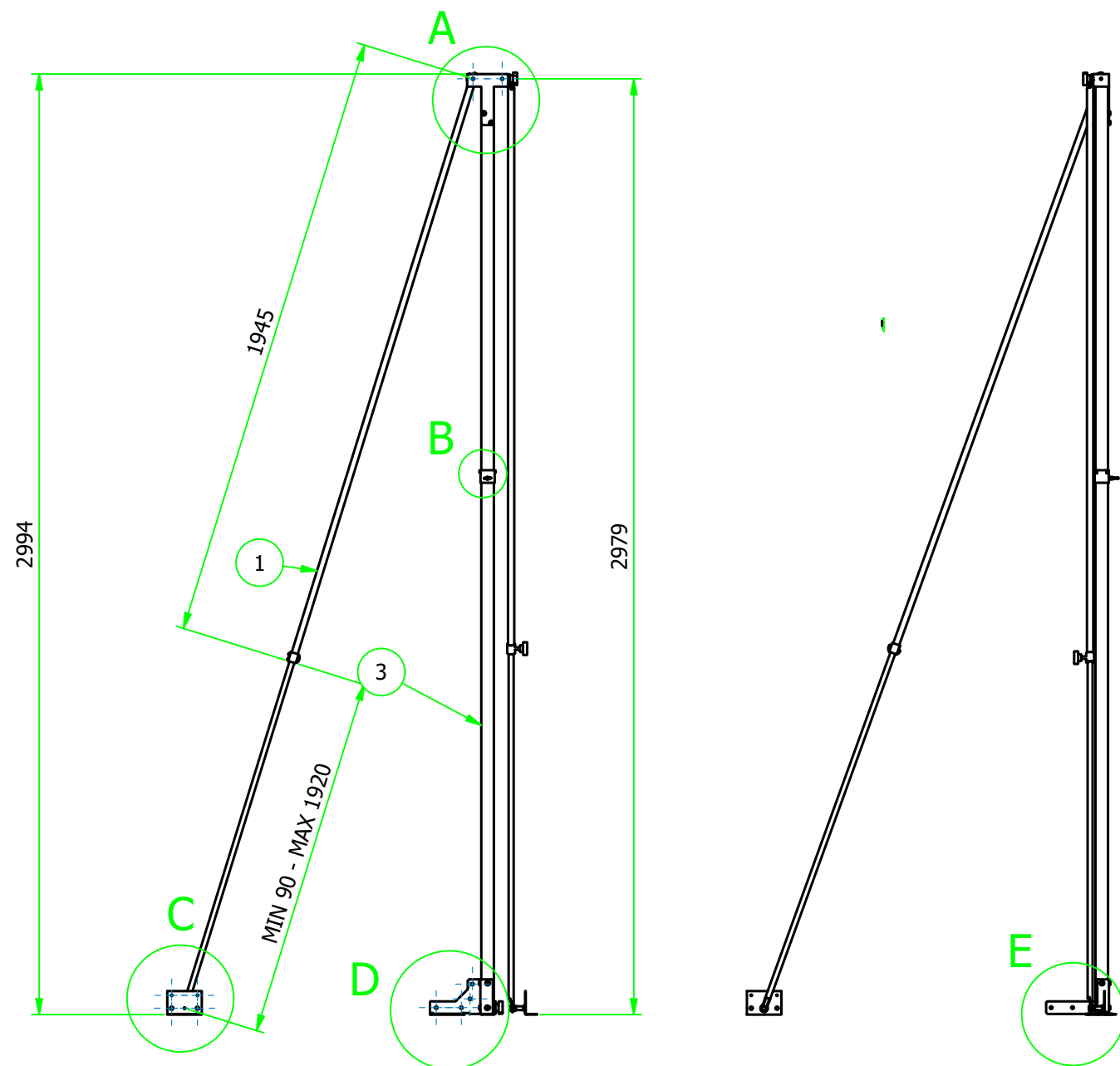
Dettaglio C Scala 1 : 5
