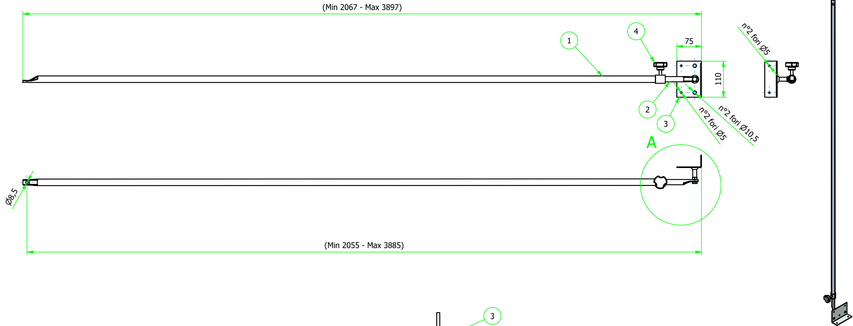
Dettaglio A Scala 1:1,5
