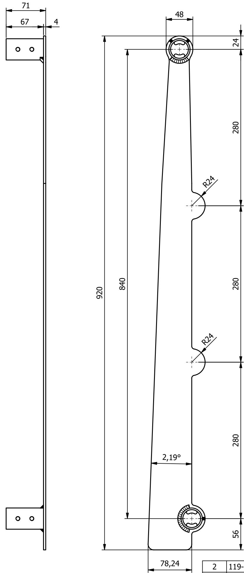
Dimensioni cod. 119-30Z
