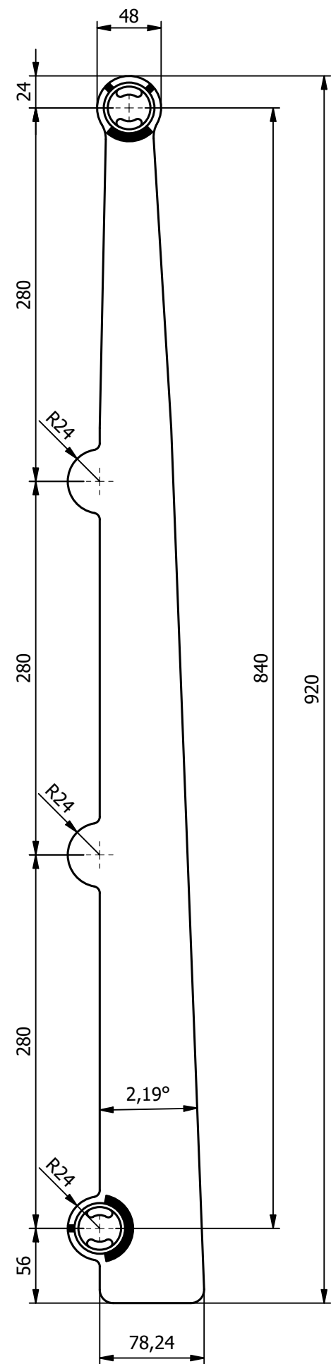
Dimensioni cod. 119-29Z
